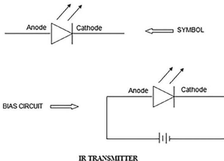
Fig. 4 IR transmitter
